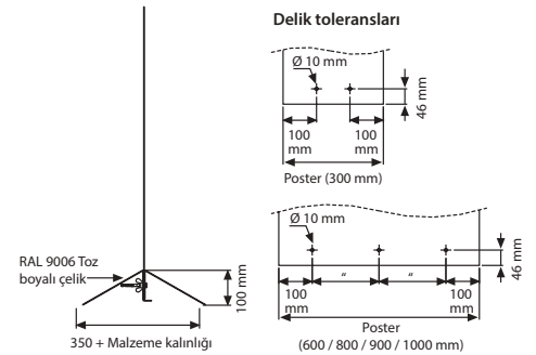
Delik toleransları
